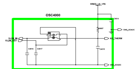
19.2MHz OSC
